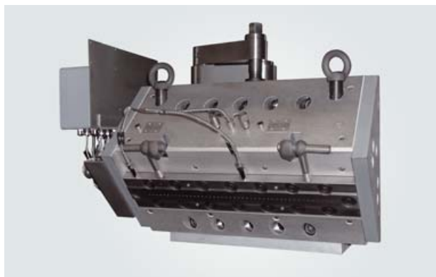
Stranggießer SG 450C
